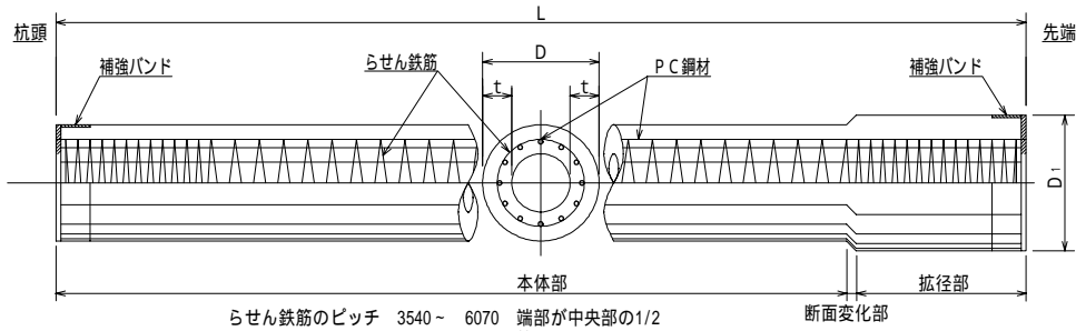
らせん鉄筋のピッチ 3540 - 6070 7080 - 110120 端部が中央部の1/2 等間隔 断面変化部
